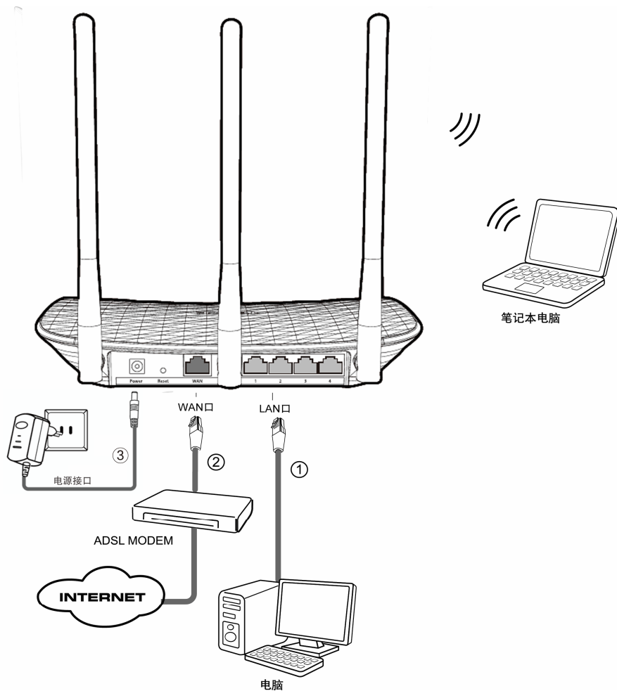
图 4-1 TL-WDR5300 硬件安装示意图
